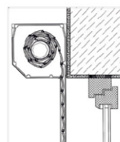
Typ „C” Roleta zamontowana na ścianie budynku (levoskrętna).
