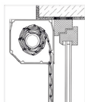
Typ „B” Roleta zamontowana we wnęcie okna (lewoskrętna).
